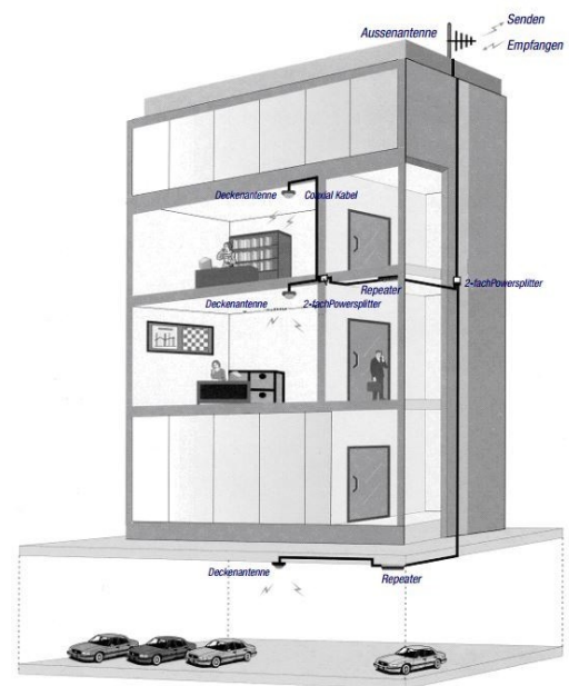
Beispiel eines Mobile Inhouse Versorgungssystems
